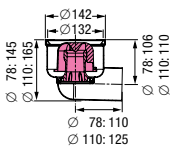
Ø 110 Art. no. 54 420
